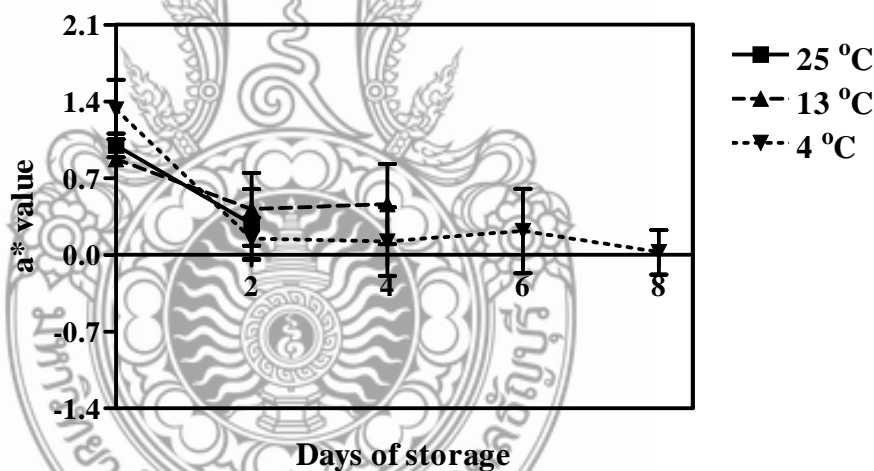
รูปที่ 4.12 ค่า a^* ของลองกองแปรรูปพร้อมบริโภคในโดยวัยที่ 1 ลองกองสุกร้อยละ 65-75 ความชื้นสัมพัทธ์ร้อยละ 90-95 เก็บรักษาที่อุณหภูมิ 4 13 และ 25 องศาเซลเซียส
