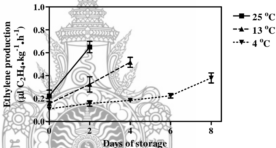
รูปที่ 4.17 อัตราการผลิตเอทิลีนของลองกองแปรรูปพร้อมบริโคนในวัยที่ 1 ลองกองสุกร้อยละ 65-75 ความชื้นสัมพัทธ์ร้อยละ 90-95 เก็บรักษาที่อุณหภูมิ 4 13 และ 25 องศาเซลเซียส
