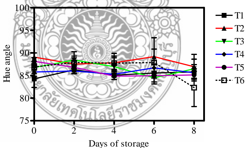
รูปที่ 4.26 ค่า Hue angle ของลองกองแปรรูปพร้อมบริโคมที่จุ่มด้วยสารละลายโซเดียมไฮโปคลอไรด์ ความเข้มข้น 0 ppm เป็นเวลา 1 นาที (T1) 100 ppm เป็นเวลา 1 นาที (T2) 200 ppm เป็นเวลา 1 นาที (T3) 0 ppm เป็นเวลา 5 นาที (T4) 100 ppm เป็นเวลา 5 นาที (T5) 200 ppm เป็นเวลา 5 นาที (T6) เก็บรักษาที่อุณหภูมิ 20 องศาเซลเซียส
